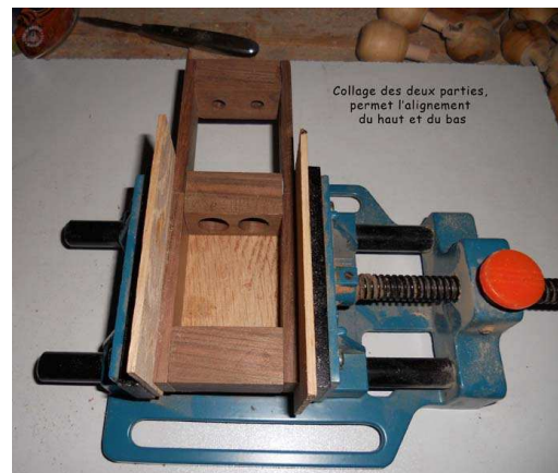
Figure 4 et 5 - Collage des deux parties. (la photo de droite montre une possibilité de collage avec l'alignement des deux parties)
