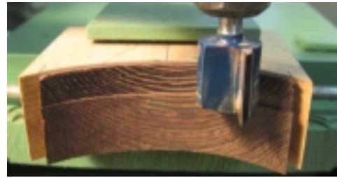
13/ Fraisage des inserts
